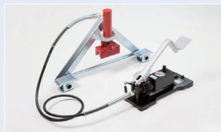
足踏式油圧ベンダー
